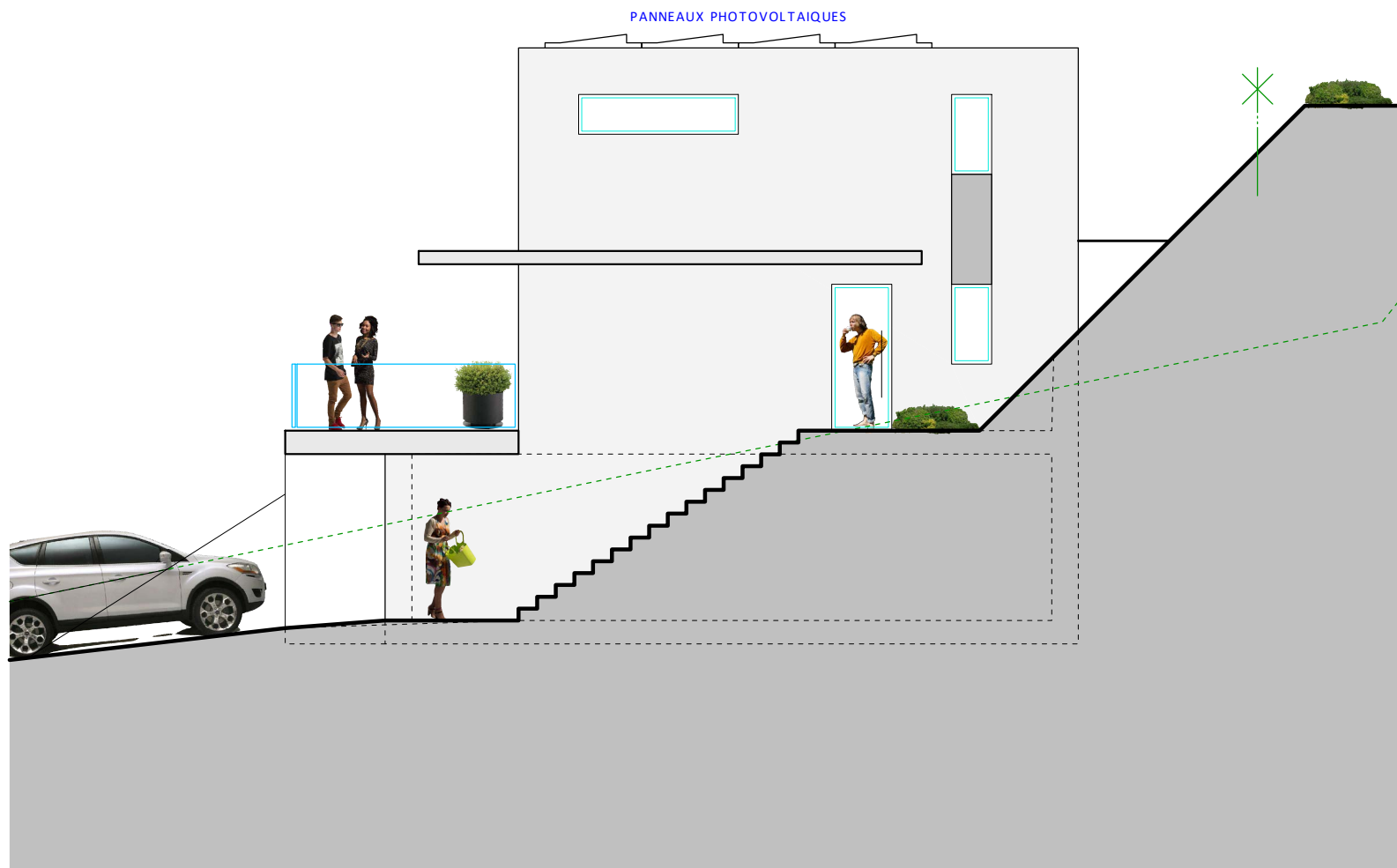
FACADE EST - 1/100
