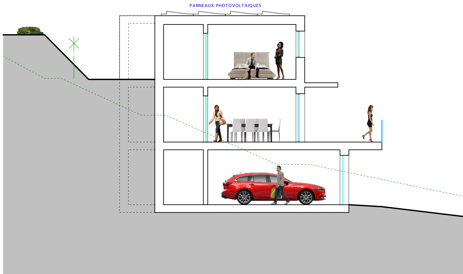
COUPE AA - 1/100
