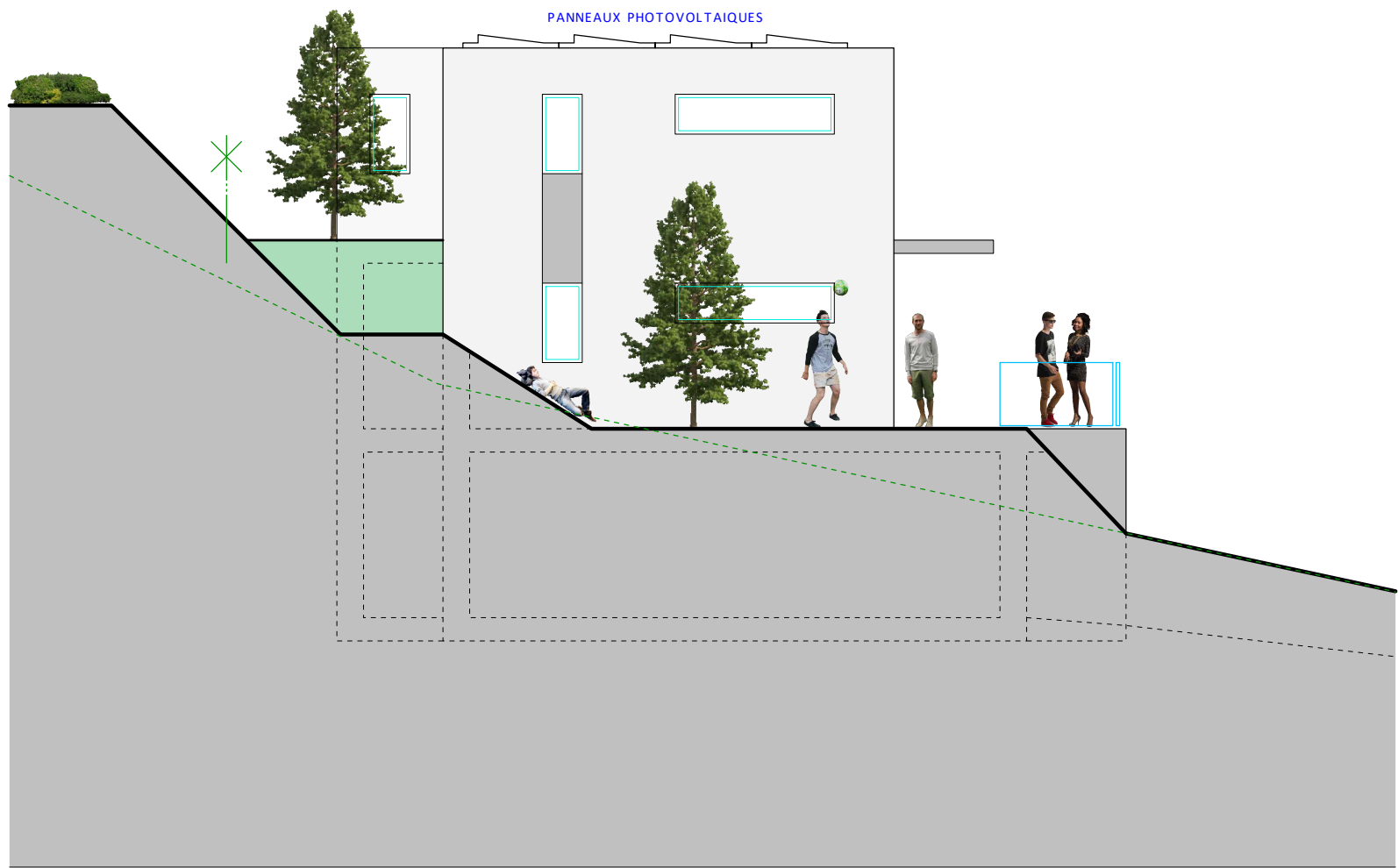
FACADE OUEST - 1/100
